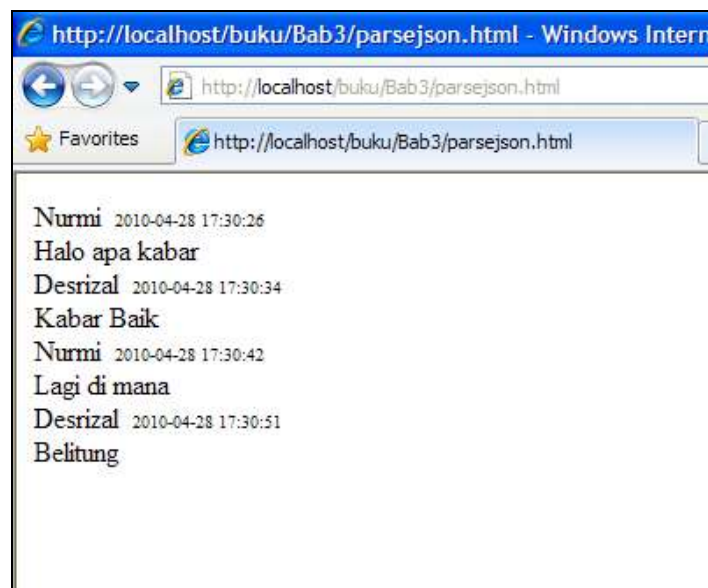
Gambar 5. Tampilan parsejson.html
