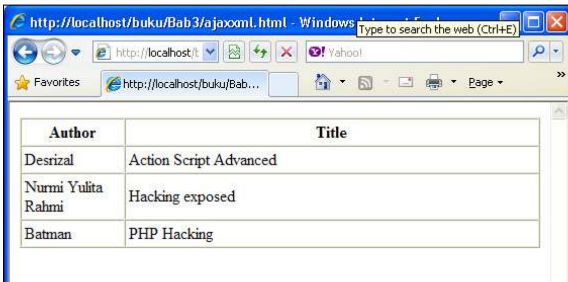
Gambar 9. Tampilan ajaxxml.html
